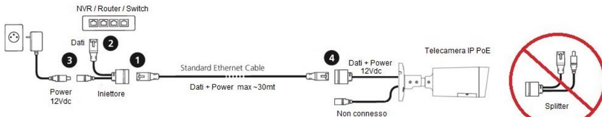
Schema di collegamento con telecamere IP LIFE cod. 75.IP080100T; 75.IP040100T2; 75.IP054100T
