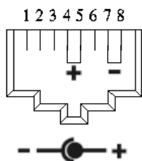
Schema di collegamento con telecamere IP LIFE cod. 75.IP080100T; 75.IP040100T2; 75.IP054100T
