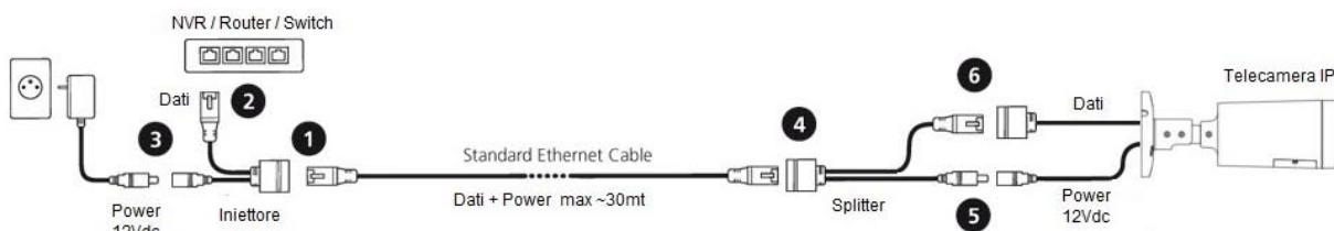
Schema di collegamento altre applicazioni es. Router/Access Point
