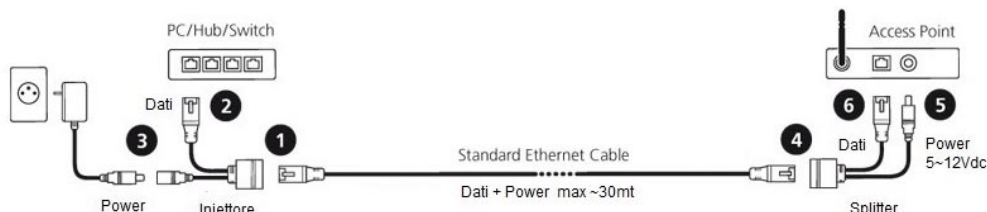
Schema di collegamento altre applicazioni es. Router/Access Point
